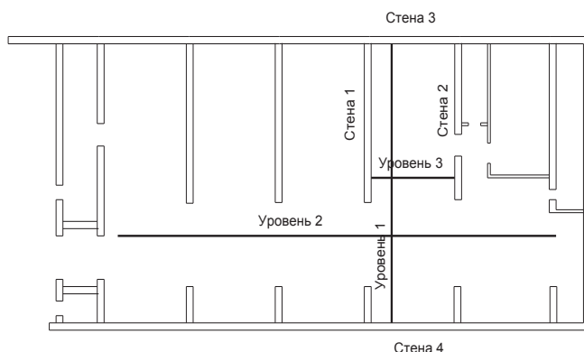
Рисунок 1 – Схема геодезических измерений элементов здания
