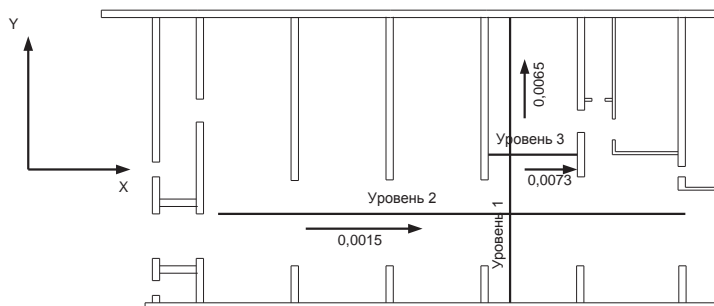
Рисунок 2 – Схема направления и величины уклонов горизонтальных уровней по перекрытию
