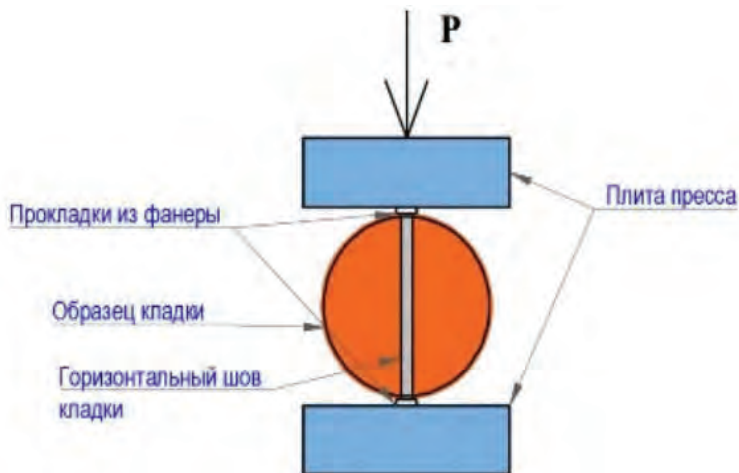
Рисунок 1 – Испытание образца
