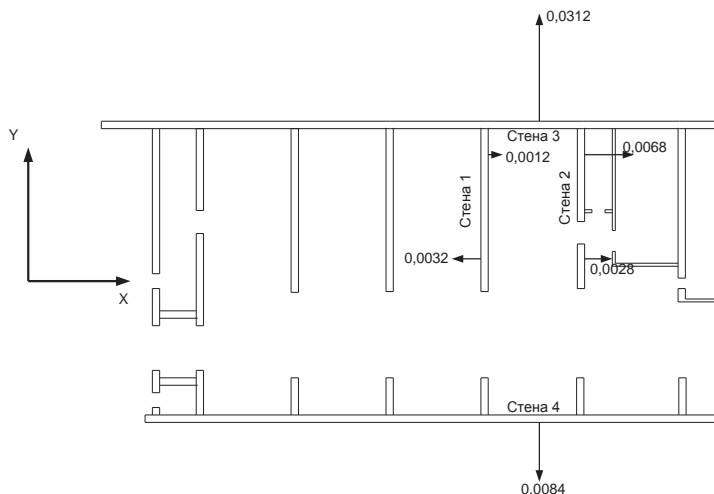
Рисунок 3 – Схема направления и величины кренов стен
