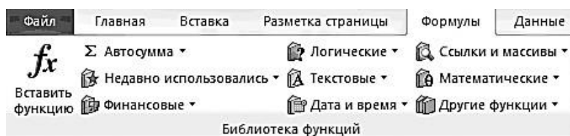
Рис. 1.1. Библиотека функций
