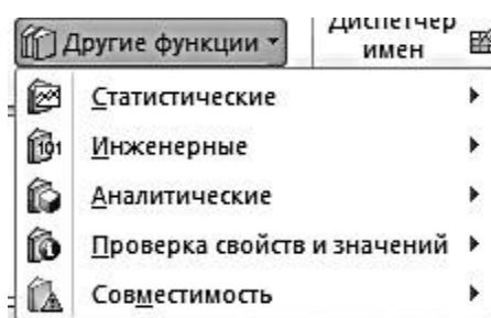
Рис. 1.2. Другие функции
