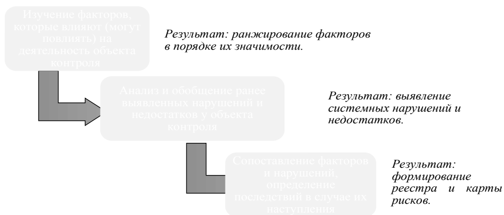
Рис. 3.2. Порядок применения риск-ориентированного подхода на подготовительном этапе проведения контрольного (экспертно-аналитического) мероприятия 8
